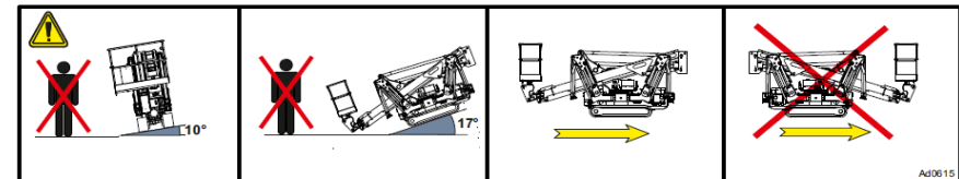
Figure 45 : pentes maximales pour la translation.
